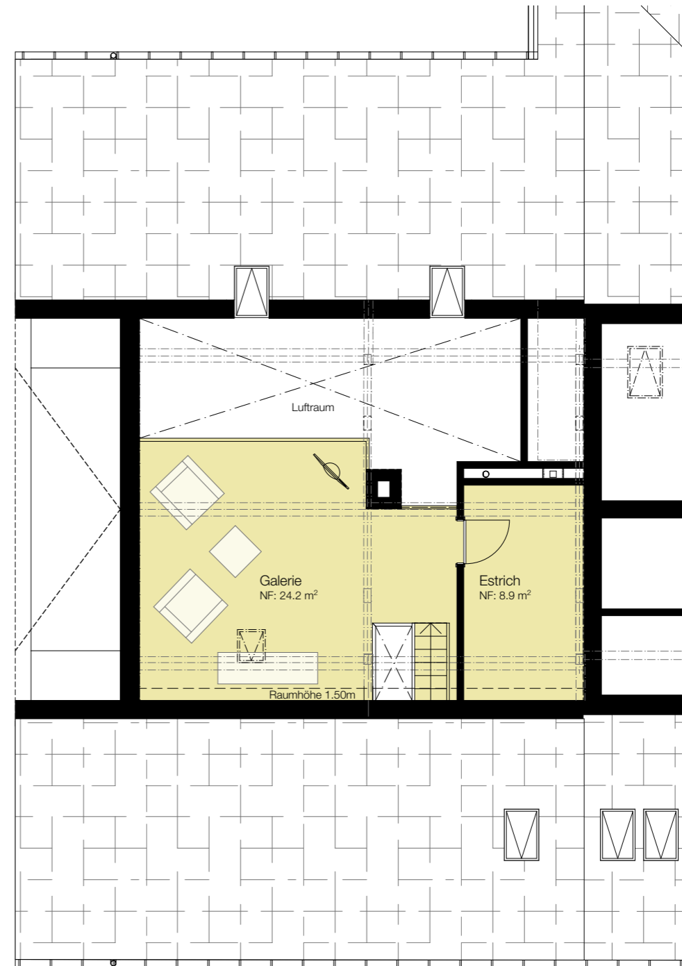
Dachgeschoss
