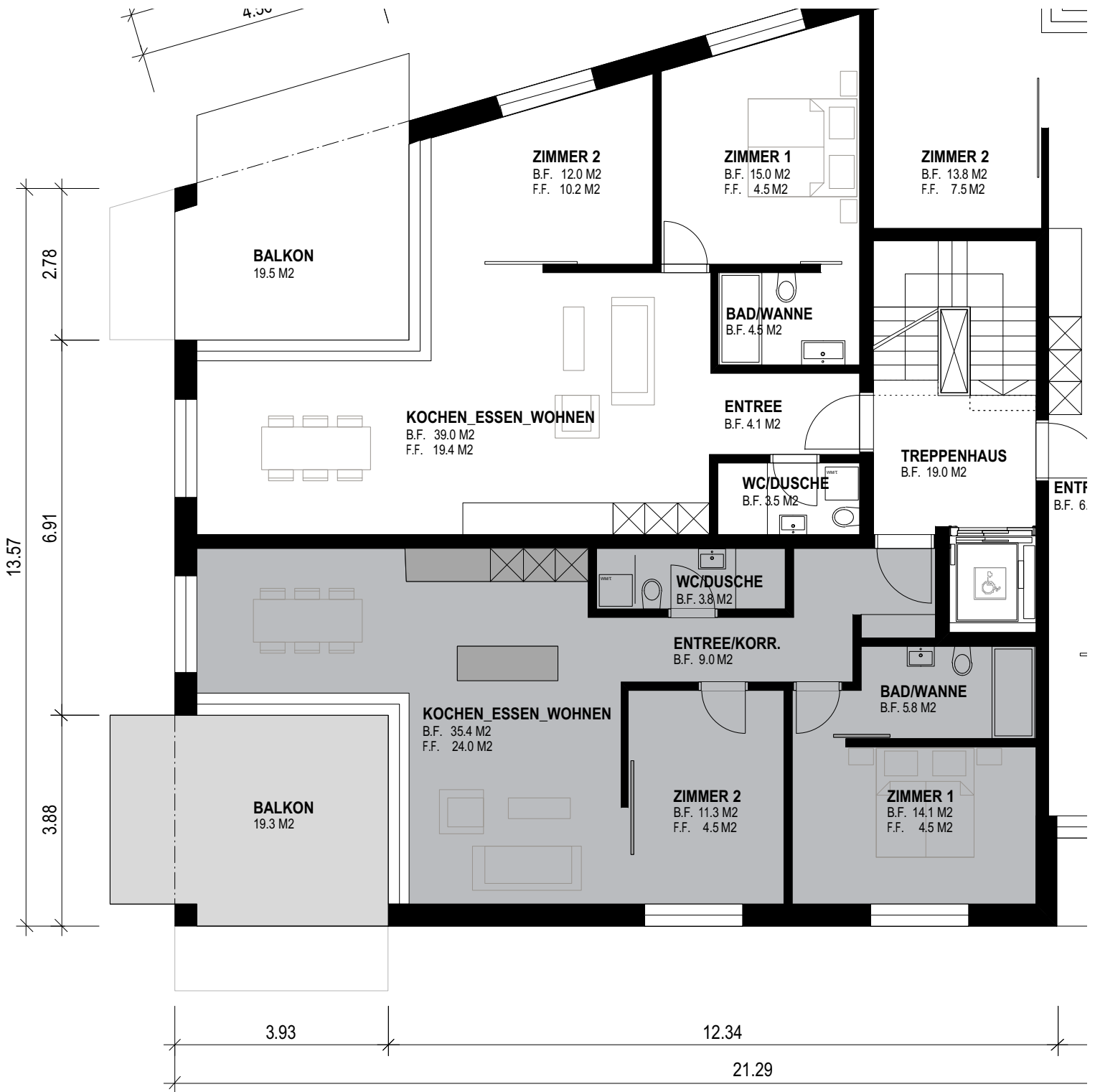
Wohnung D.05 3 1/2 - ZIMMER BGF 94.8 M2
