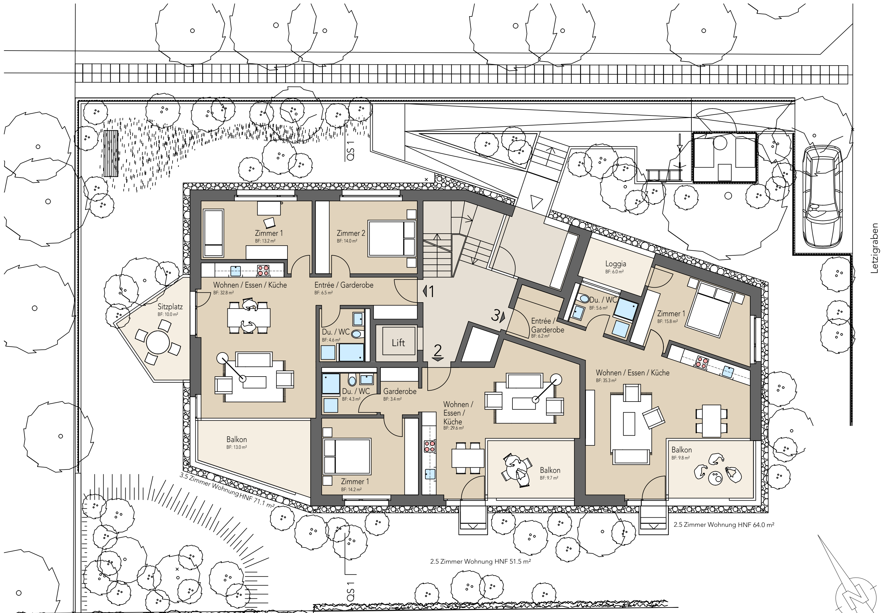
Erdgeschoss Letziggraben 126
