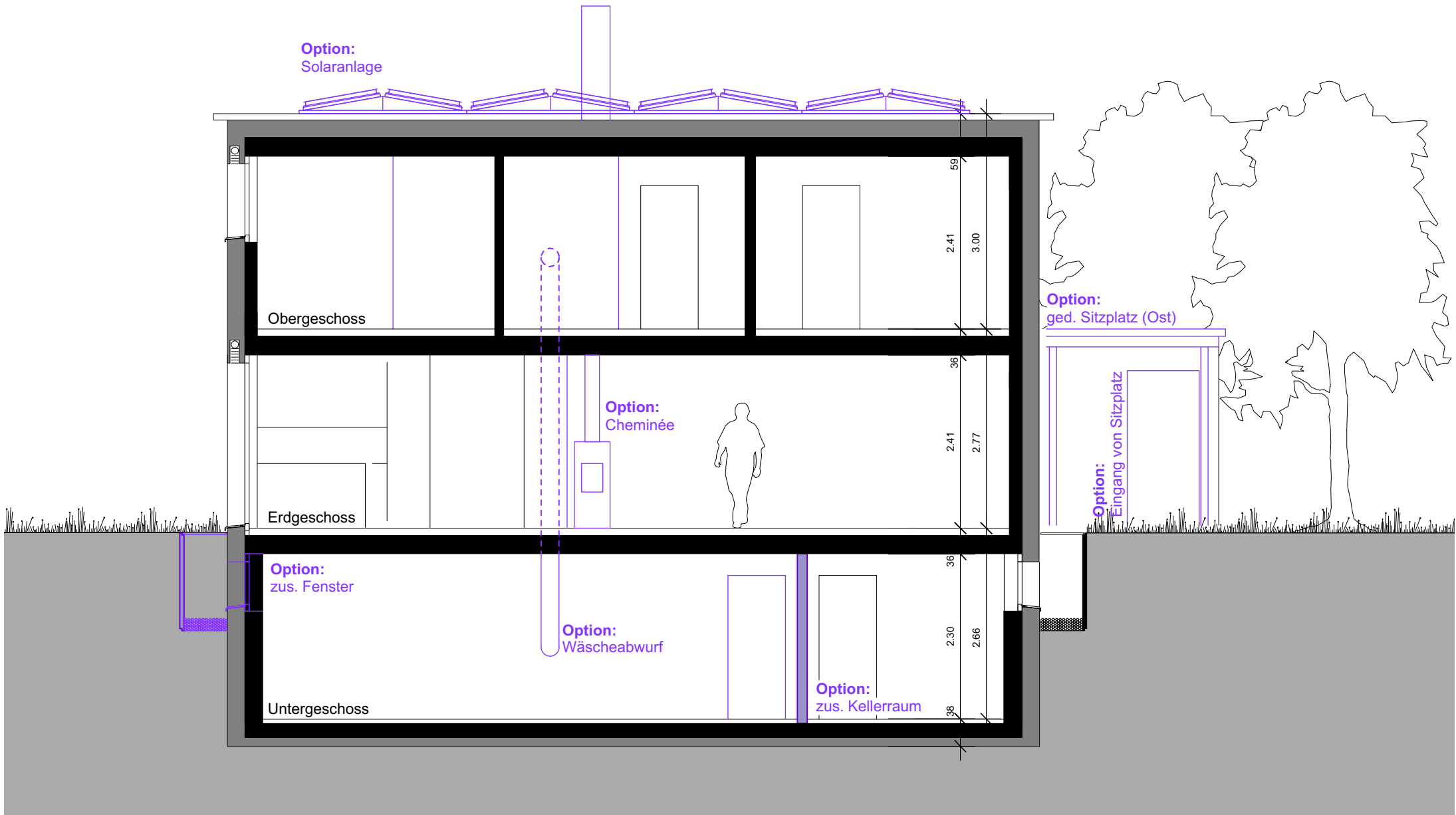
Längsschnitt
